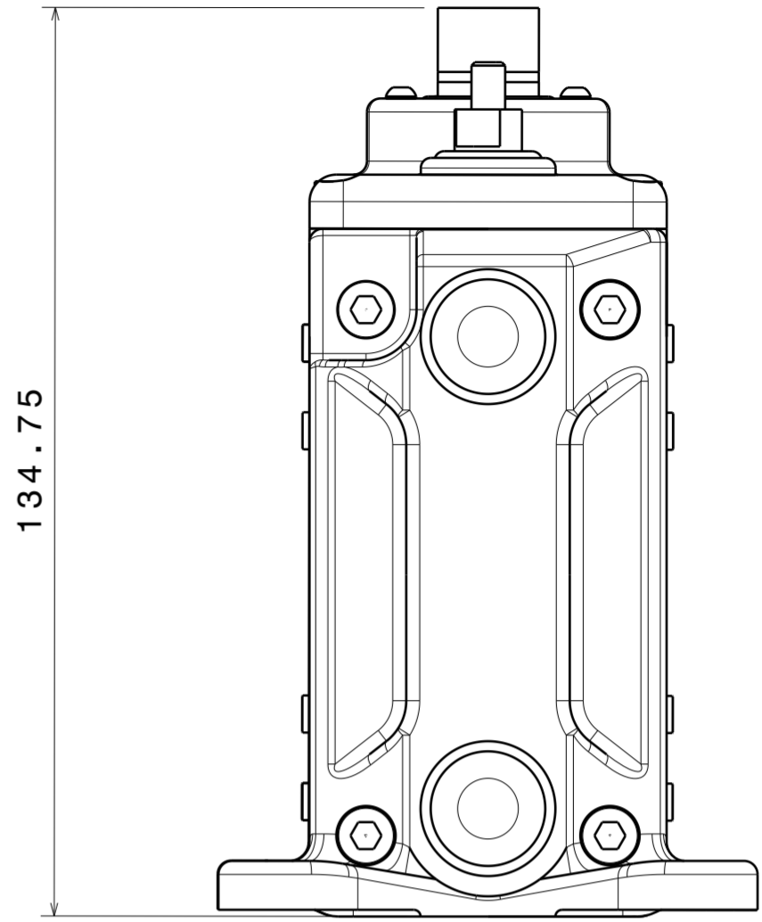
Vue de gauche Echelle : 1:1
